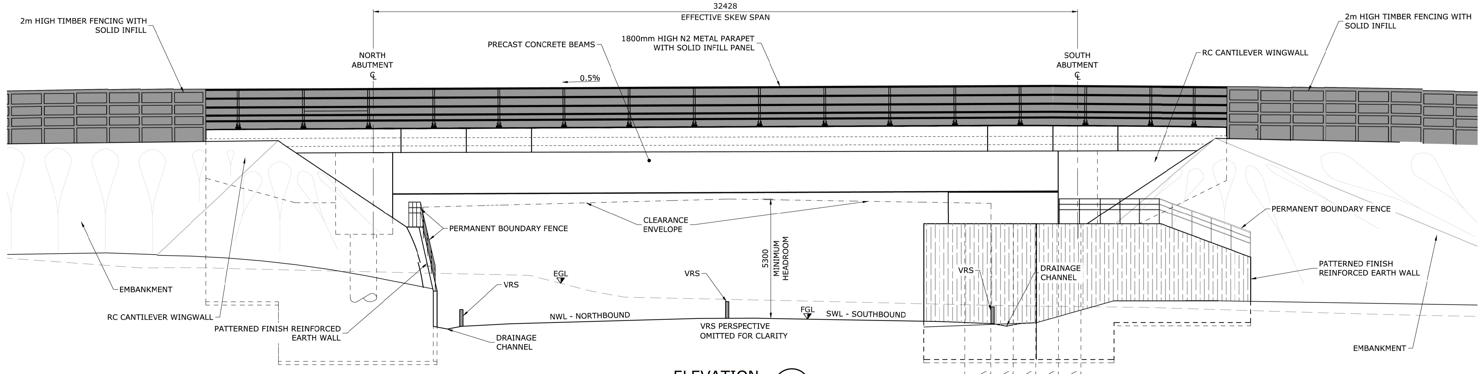
ELEVATION (A-A) 1:100
